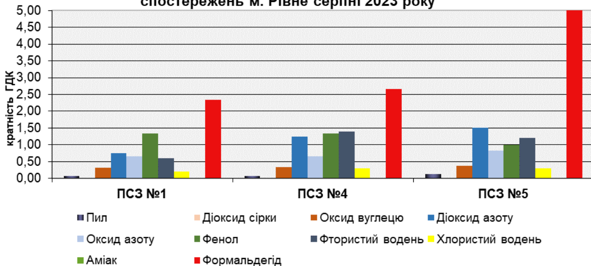
рис. 1.3. Середньомісячні концентрації (в кратності середньодобових ГДК) забруднюючих речовин в розрізі постів спостережень м. Рівне серпні 2023 року
