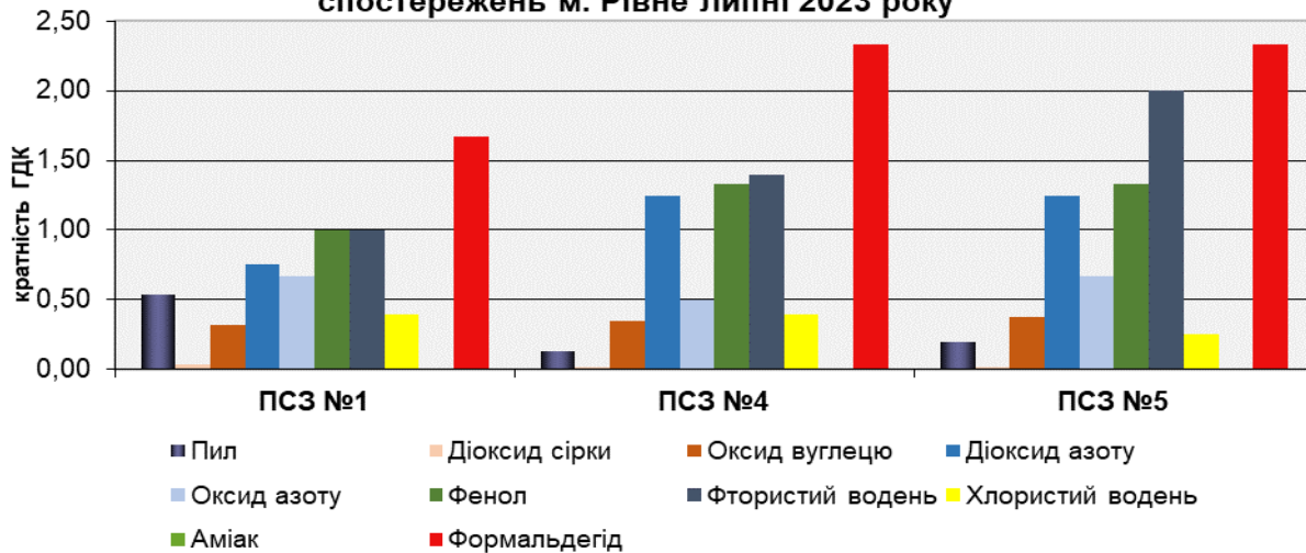
рис. 1.2. Середньомісячні концентрації (в кратності середньодобових ГДК) забруднюючих речовин в розрізі постів спостережень м. Рівне липні 2023 року
