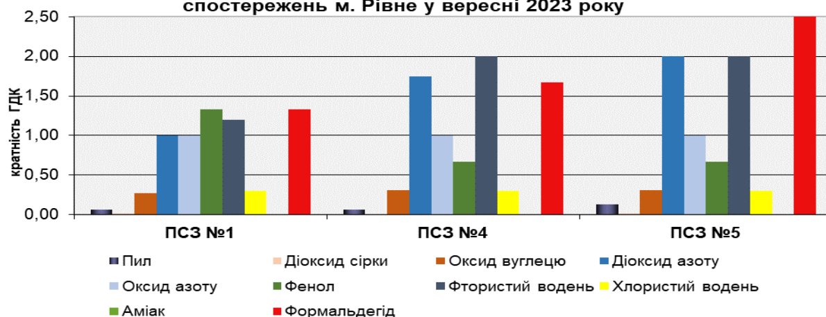
рис. 1.4. Середньомісячні концентрації (в кратності середньодобових ГДК) забруднюючих речовин в розрізі постів спостережень м. Рівне у вересні 2023 року
